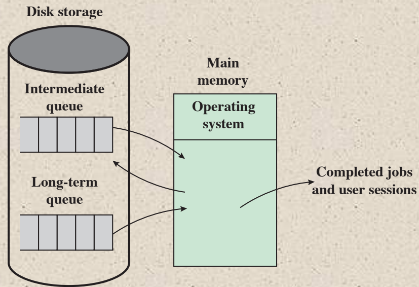
(b) Swapping
